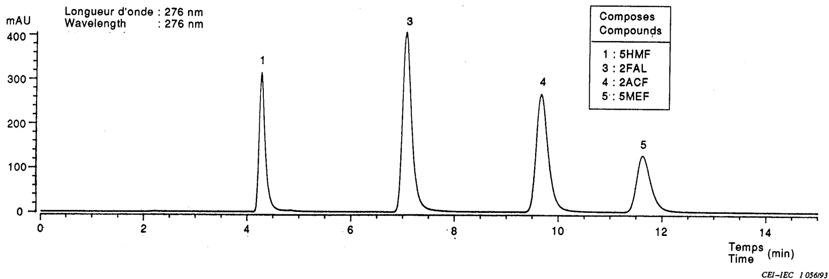
Figure 2 – Exemples de chromatogrammes enregistrés à deux longueurs d'ondes (220 nm et 276 nm) Examples of chromatograms recorded at two wavelengths (220 nm and 276 nm)
